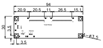
CONTROLLER SC 2:1
